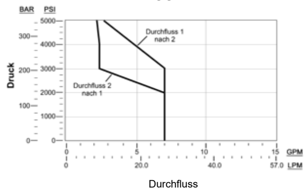
DTAF-*C* mit High-Power-Spule (In Ruhestellung geschlossen)
