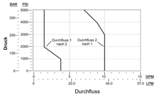
DTAF-*H* mit High-Power-Spule (In Ruhestellung offen)
