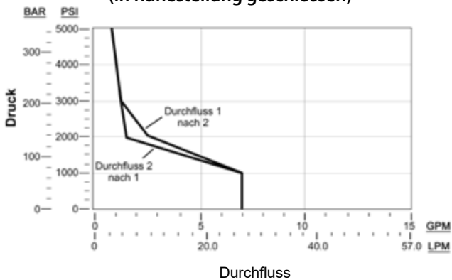
DTAF-*C* mit Low-Power-Spule (In Ruhestellung geschlossen)
