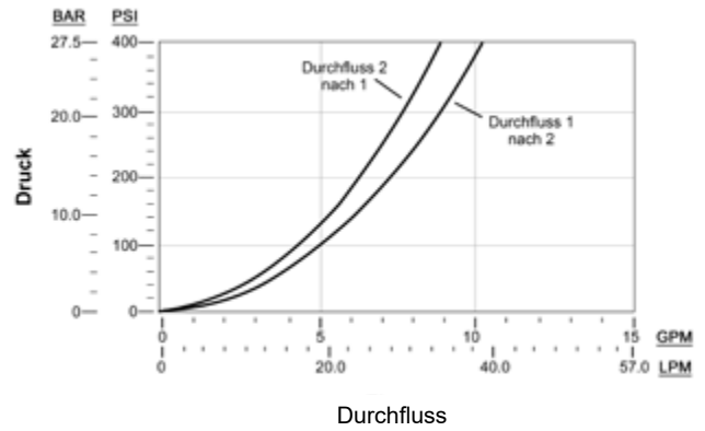
DTAF-*H* (In Ruhestellung offen)
