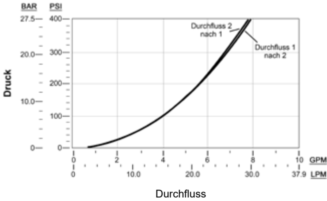
DTAF-*C* (In Ruhestellung geschlossen)
